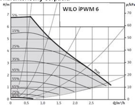
Obrázek 4.4.1 Charakteristiky čerpadla
