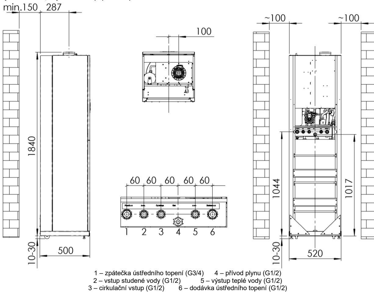
Obrázek 3.3.1 Montážní rozměry kotle
