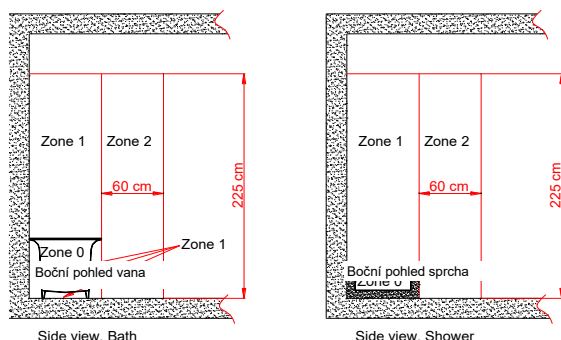
Obrázek 3.1.2.1 Rozměry zón v prostorách s vanou nebo sprchou a vaničkou
