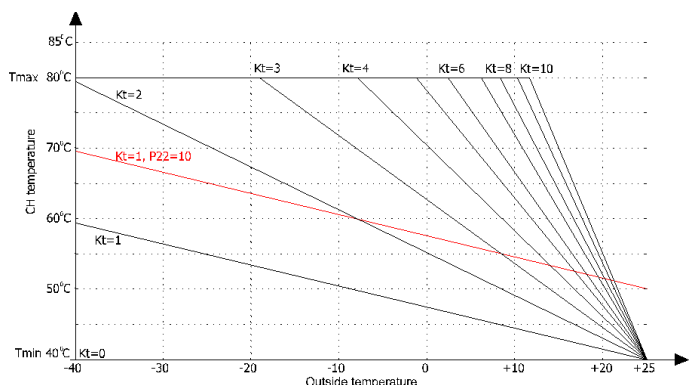
Obrázek 2.4.2.1 Diagram topné křivky (standardní topení) Obrázek 2.4.2.2 Diagram topné křivky (podlahové topení)
