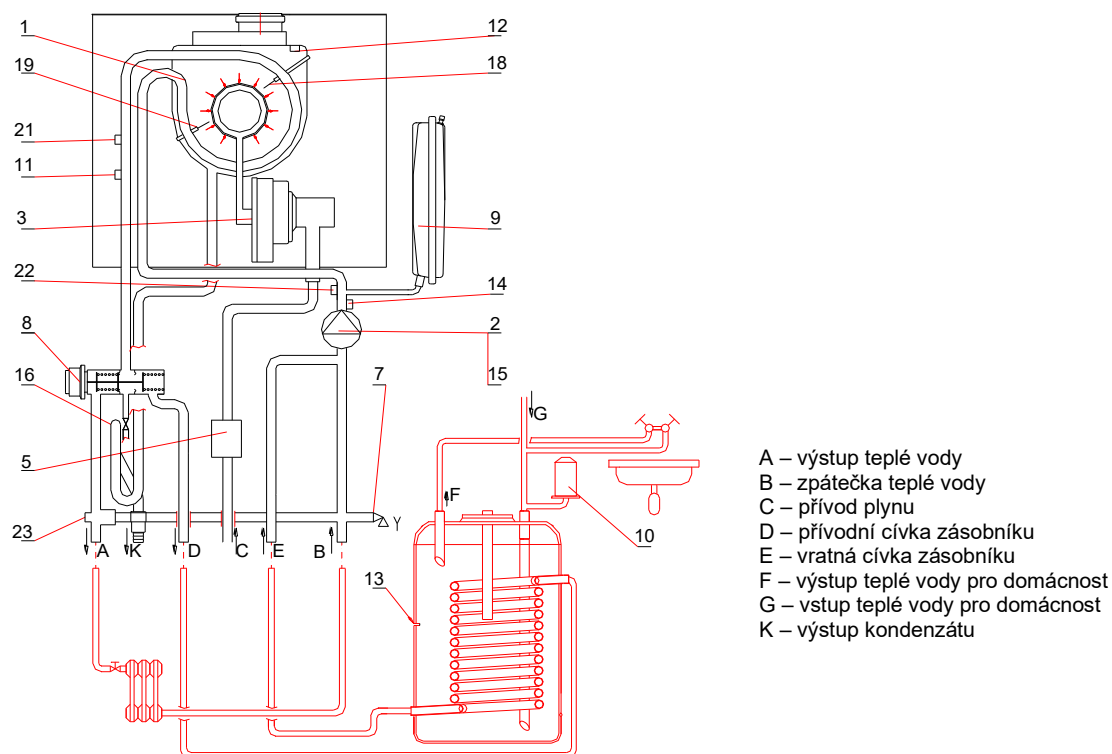
Obrázek 2.2.1.2 Schéma provozu kotle
