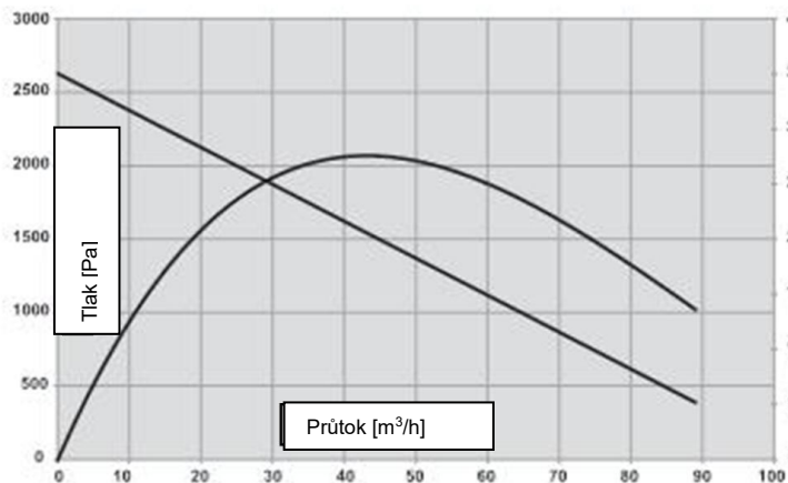
Obrázek 4.4.1 Charakteristiky ventilátoru typu PX 118
